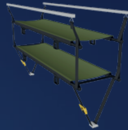
AUFNAHMESYSTEM FÜR KRANKENTRAGEN
